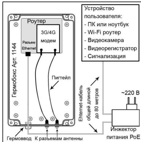
Схема 6 – Пример размещения оборудования в гермобоксе (артикул 1144, поставляется отдельно)
