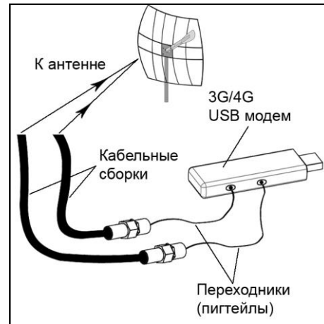
Схема 7 – Пример подключения USB модема к MIMO антенне
