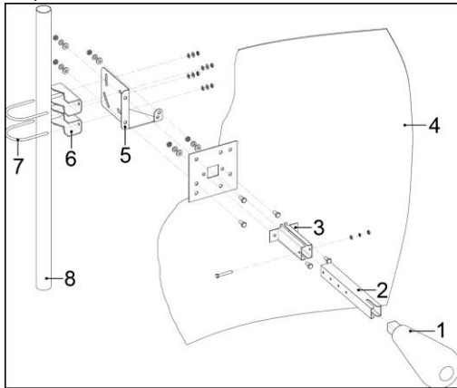
Схема 1 – Сборка антенны
