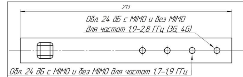
Схема 3 – Установка стойки облучателя антенны с усилением 24 дБ
