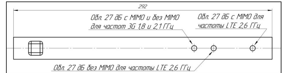
Схема 4 – Установка стойки облучателя антенны с усилением 27 дБ
