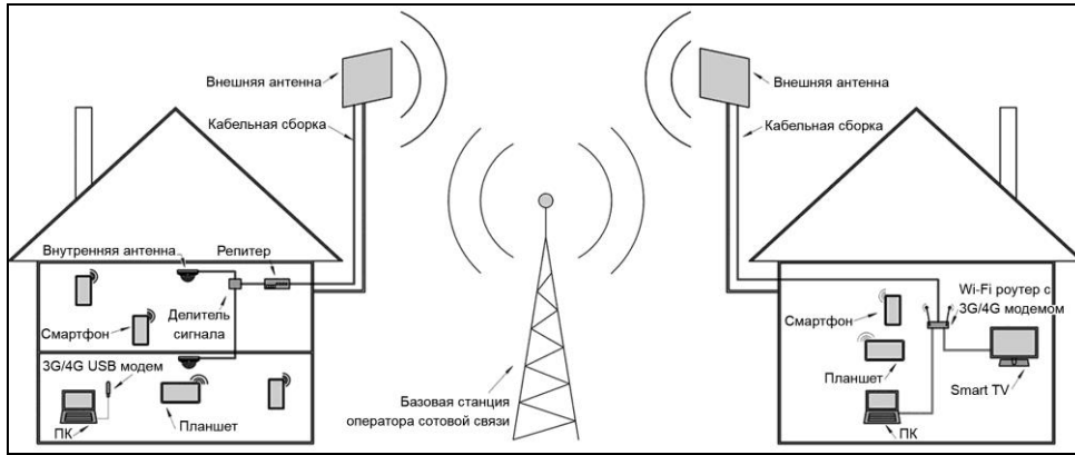
Схема 5 - Примеры установки и подключения антенны к оборудованию
